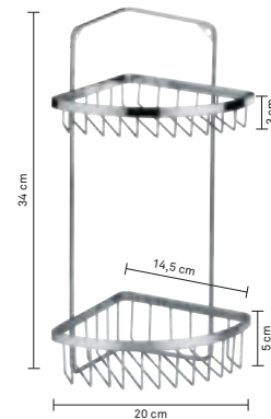
Eckregal Corner rack · Etagère d'angle
