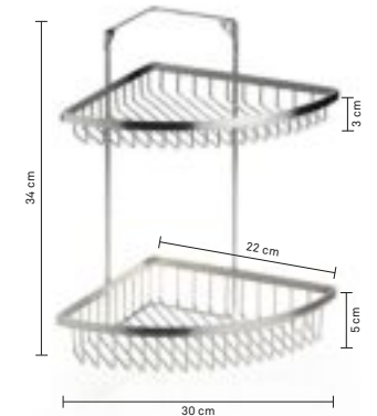
Eckregal Corner rack · Etagère d'angle
